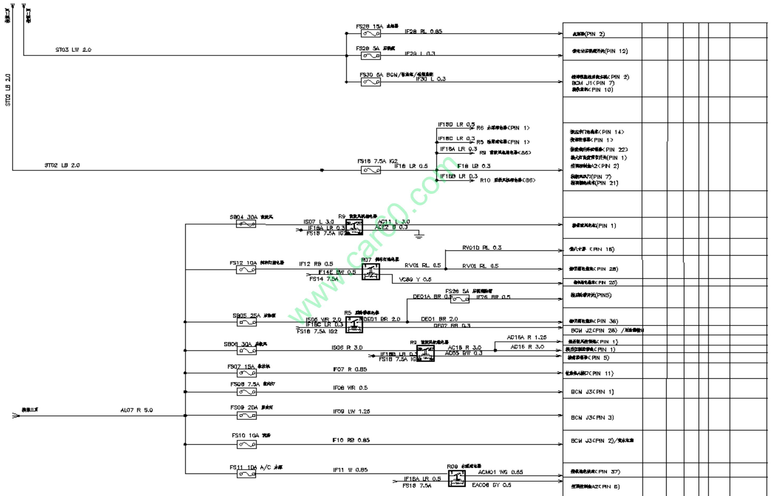
整车电源分配图
